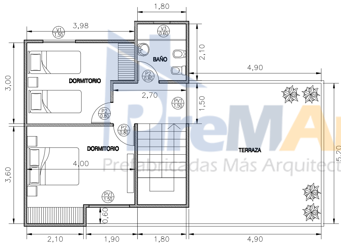
PLANTA ALTA
