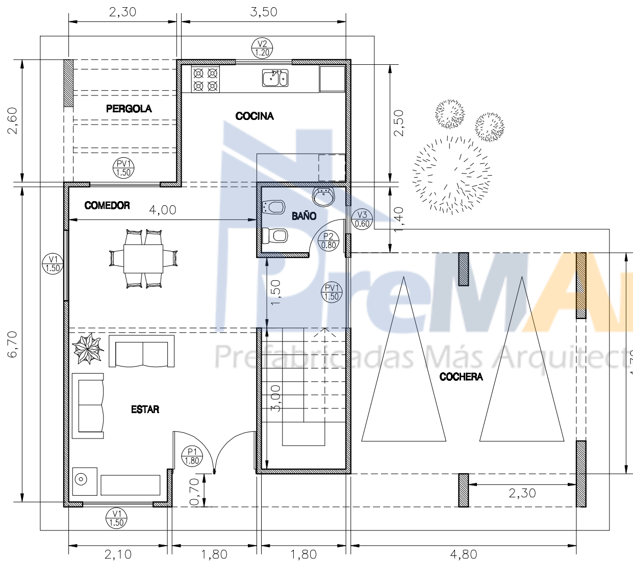
PLANTA BAJA
